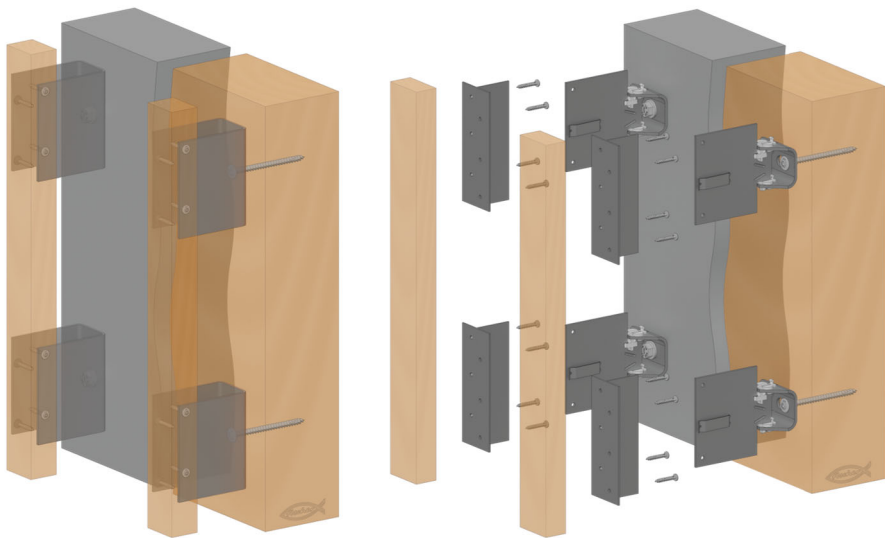
z.B. fischer BWM Fassadensystem Holzhalterung Typ H1 z.B. fischer BWM Fassadensystem Holzhalterung Typ T2
