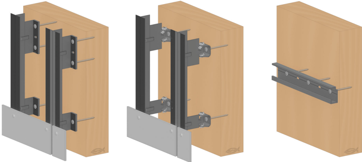
z.B. fischer BWM Fassadensystem AKT 100 z.B. fischer BWM Fassadensystem AKT 100 Zela z.B. fischer BWM Fassadensystem AKT 103
