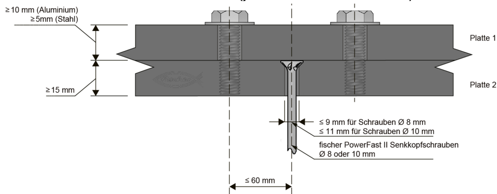
Abbildung L1.1: Schraubenkopf Stützplatten für fischer PowerFast II Schrauben (Abbildung nicht maßstäblich)
